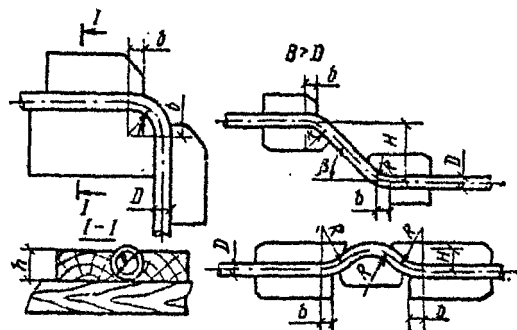
Рис. 18. Шаблоны для получения гнутых деталей
