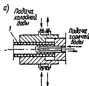
Рис. 16. Схема формирования отбортовки
