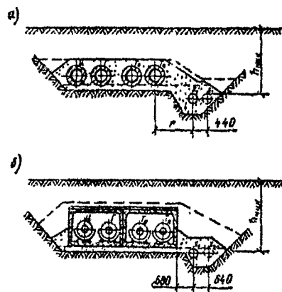
Рис. 9. Схемы совмещенной прокладки пластмассовых трубопроводов:
