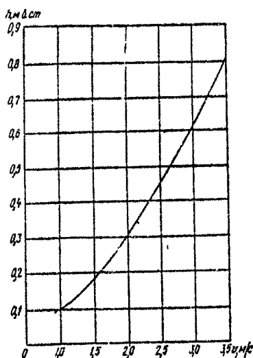
Рис. 7. Потери напора в односегментном крене
