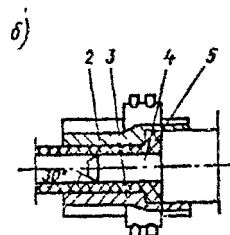
Рис. 17. Схема формирования утолщенного бурта на конце трубы
