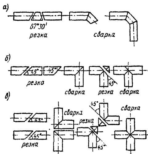
Рис. 22. Схема процесса изготовления фасонных частей контактной стыковой сваркой а — отводы и колена, б — тройников; в — крестовины
