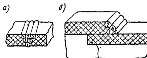
Рис. 21. Порядок укладки сварочных прутков в шов а — при стыковом соединении, б — при соединении в рывтуб
